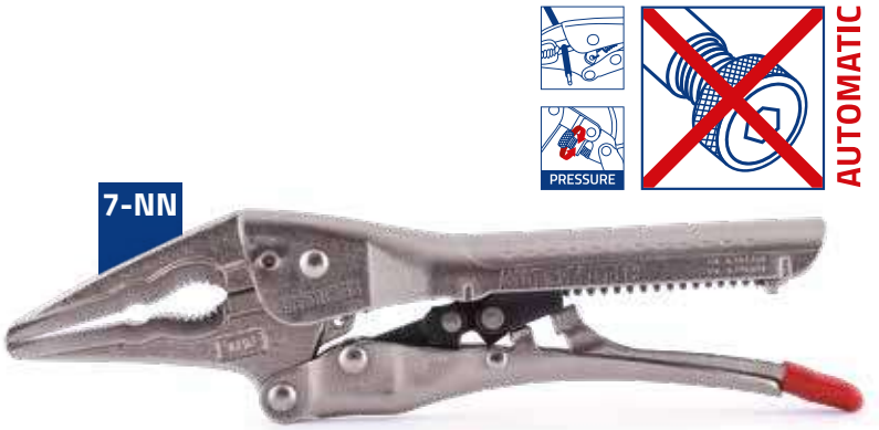
Automatic long nose locking plier with wire cutter Automatische puntgriptang met draadknipper Pince-étau automatique, becs longs avec coupe-câble
